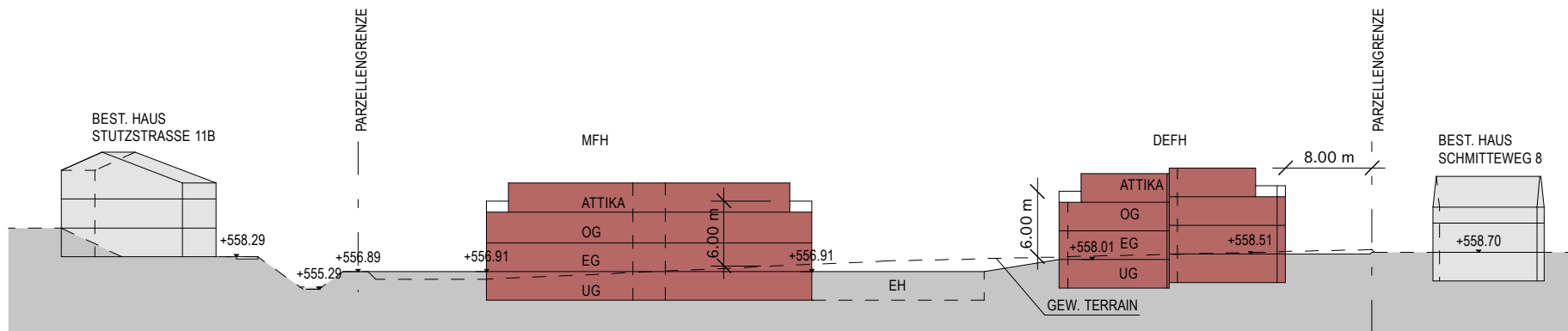
SCHNITT SÜD - NORD (B - B)
